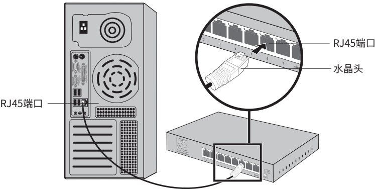
图3-1 RJ45端口连接示意图
