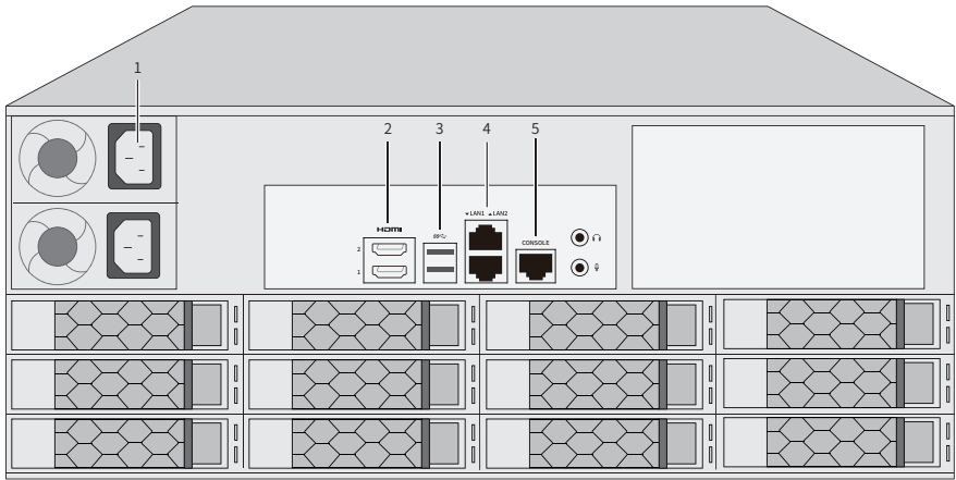
图1-3 TL-NVS7362-256后面板示意图
