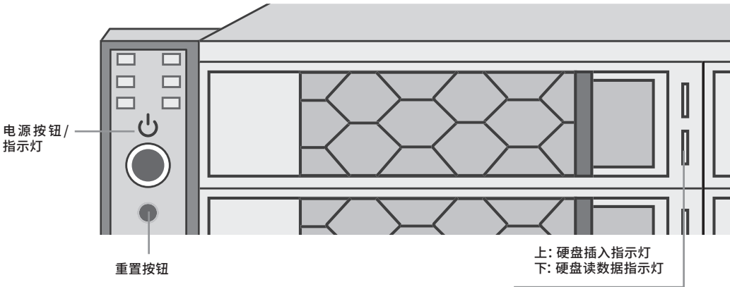
图1-2 前面板按钮与指示灯
