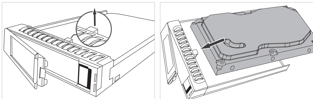
图3-3 安装硬盘
