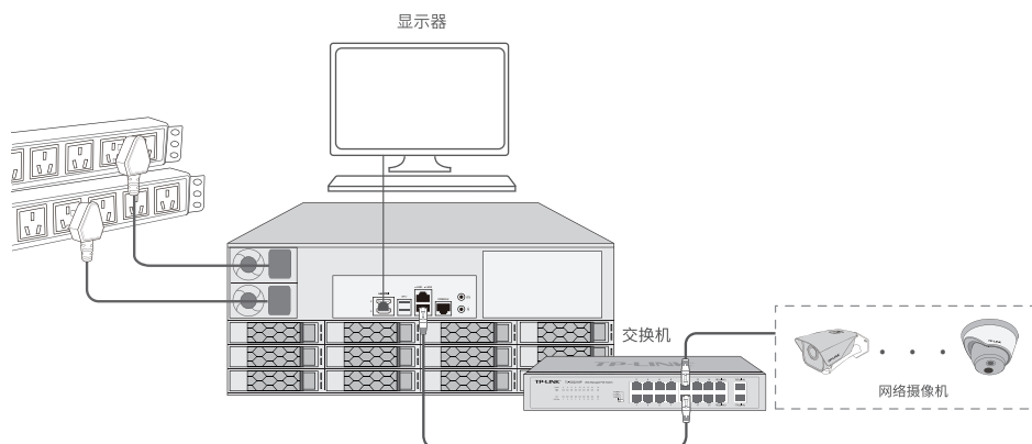
图3-6 单机状态NVS连接示意图
