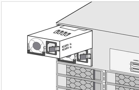
图3-1 安装电源模块
