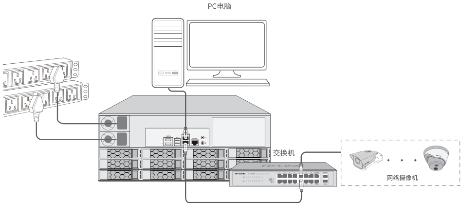
图3-4 NVS连接示意图
