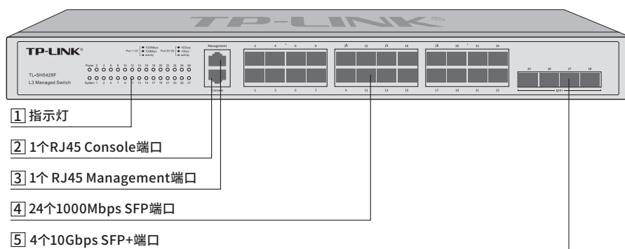
图1-3 TL-SH5428F前面板示意图
