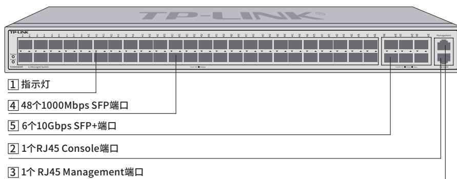
图1-4 TL-SH5654F前面板示意图
