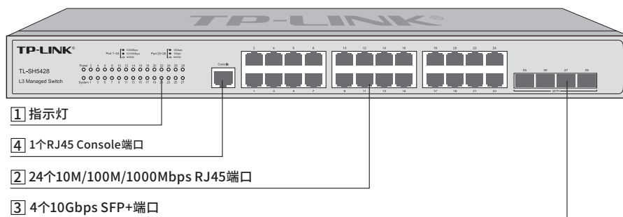
图1-1 TL-SH5428前面板示意图
