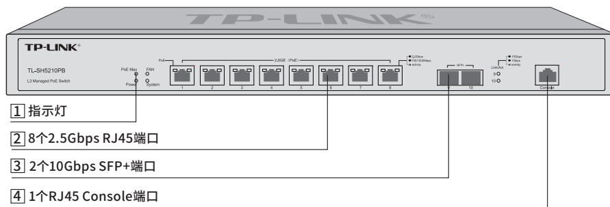
图1-6 TL-SH5210PB前面板示意图
