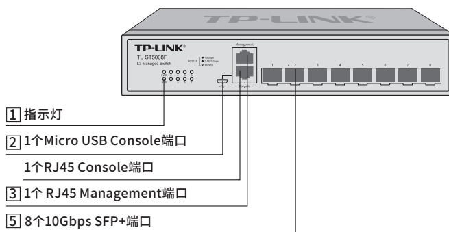
图1-5 TL-ST5008F前面板示意图
