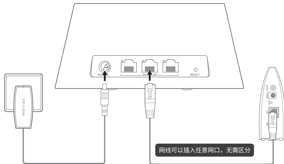
POWER接口： 连接配套的电源适配器
