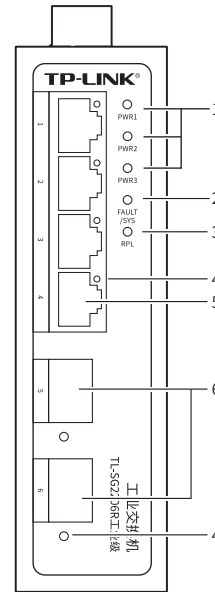
TL-SG2206R工业级 前面板示意图
