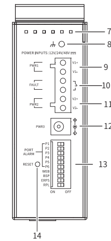
TL-SG2206R工业级 上面板示意图
