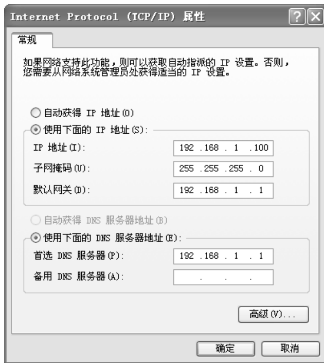
图4-1 本地连接
