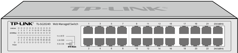
图 2-5 TL-SG2024D前面板
