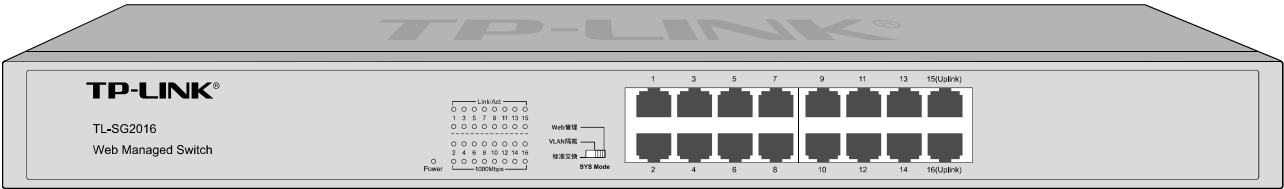
图 2-4 TL-SG2016前面板
