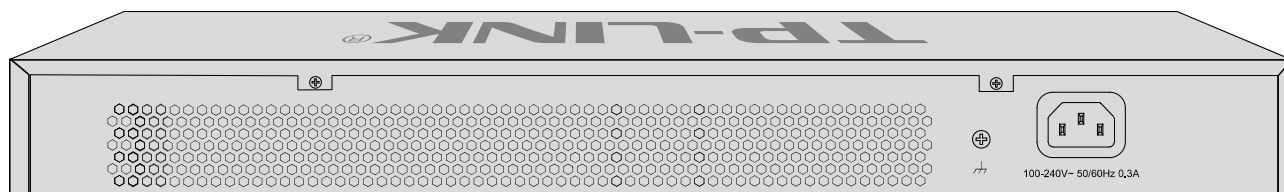
图 2-8 后面板
