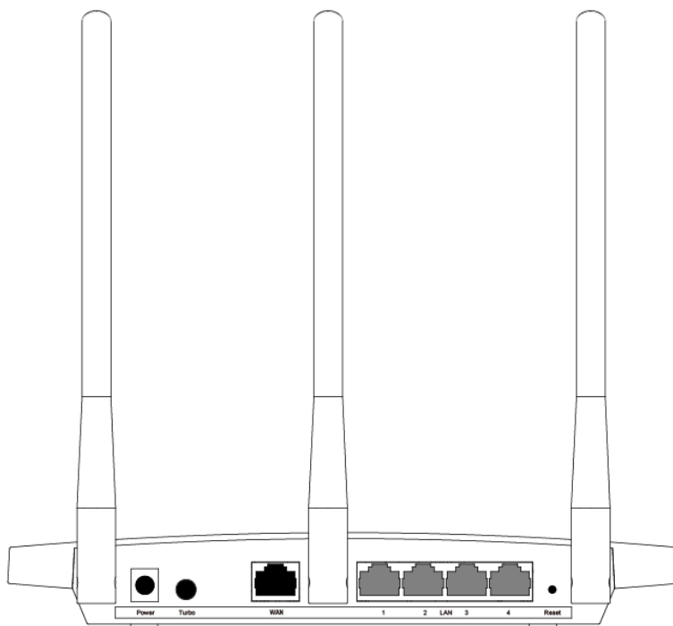
图 3-2 TL-WR2041N 后面板示意图
