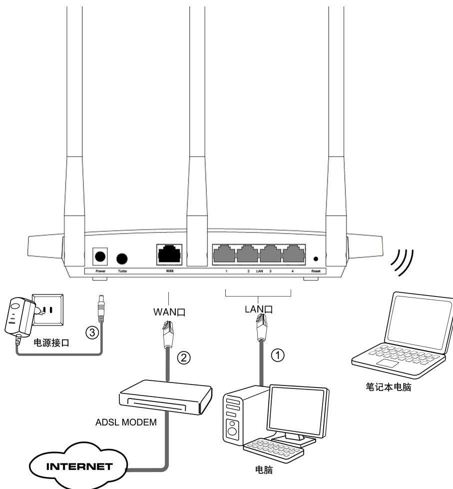
图 4-1 TL-WR2041N 硬件安装示意图
