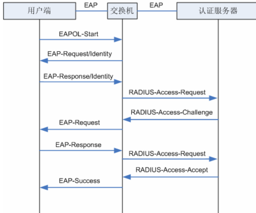
图 12-18 EAP-MD5 认证过程
