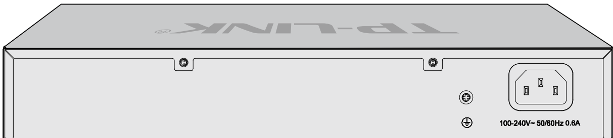
图 2-5 后面板（以 TL-SG3210 为例）
