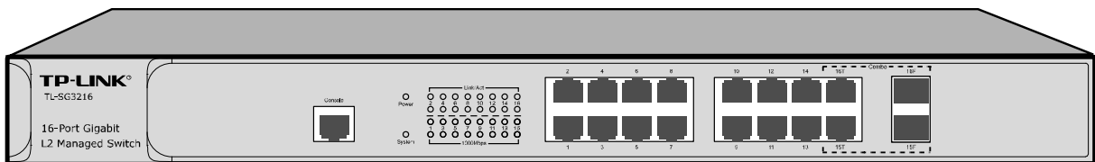
图 2-3 TL-SG3216 的前面板
