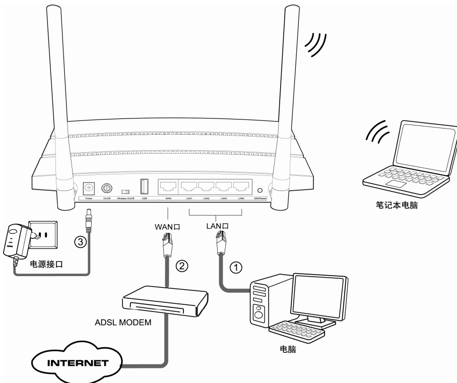
图 4-1 TL-WDR3300 硬件安装示意图
