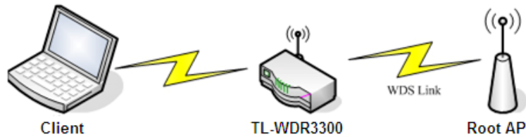
图 5-27 WDS 连接拓扑图
