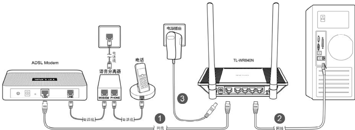
图 4-1 TL-WR840N 硬件安装示意图
