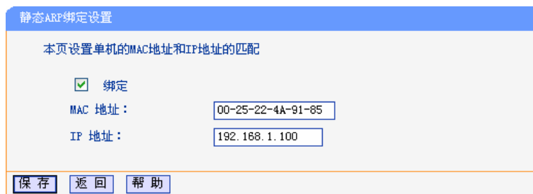
图 5-44 添加静态 ARP 绑定条目
