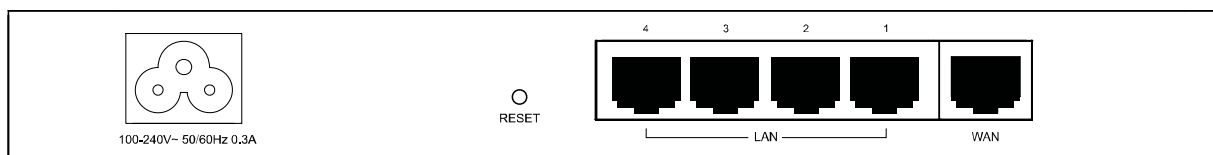
图 2-8 TL-R473 后面板示意图
