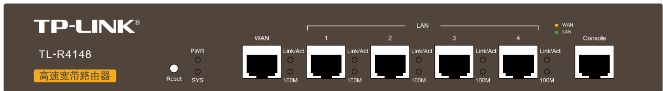
图 2-5 TL-R4148 前面板示意图
