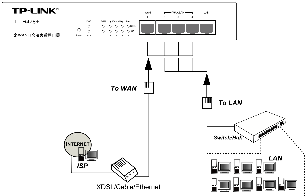
图 3.3 建立局域网和广域网连接
