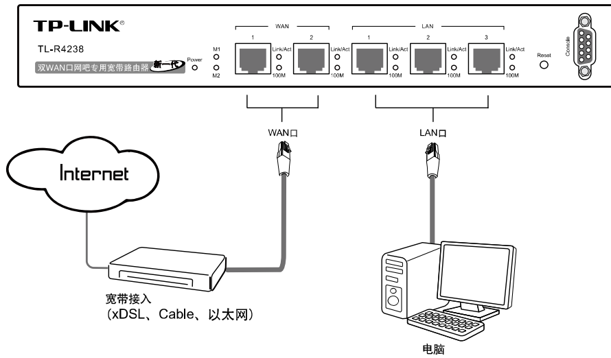
图 3.7 建立局域网和广域网连接
