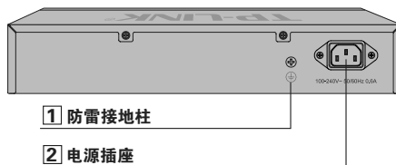
图1-2 后面板示意图
