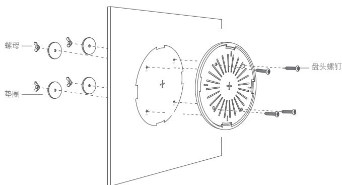
图3-4 固定安装架到天花板示意图
