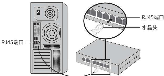
图3-1 RJ45端口连接示意图
