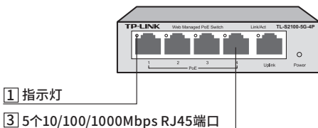
图1-3 TL-S2100-5G-4P前面板示意图
