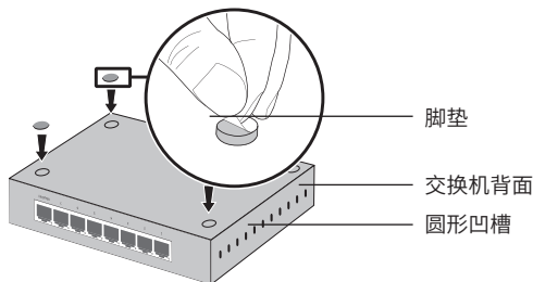
图2-1 桌面安装示意图
