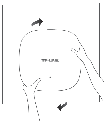
图3-13 壁挂安装完成示意图
