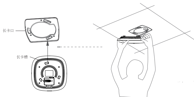
图3-6 安装AP到安装架示意图
