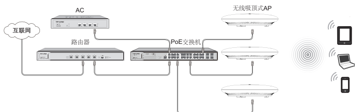
图1-4 典型应用拓扑图-FIT AP模式
