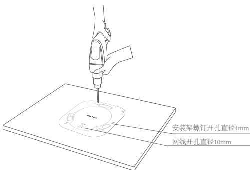
图3-3 钻孔示意图
