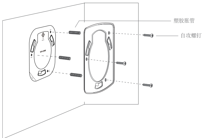
图3-11 固定安装架到墙面示意图
