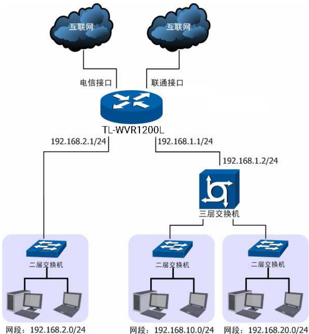
图 4-88 NAPT功能组网应用
