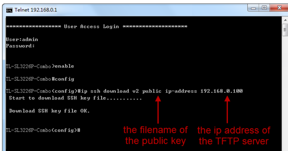
图 1-12 导入公钥文件至交换机
