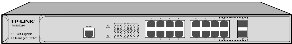
图 2-3 TL-SG3216 的前面板
