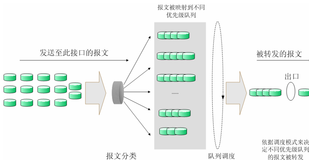
图 9-1 QoS 工作原理
