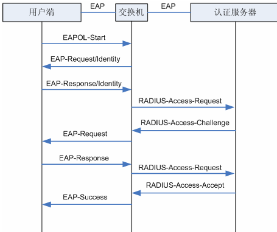
图 12-18 EAP-MD5 认证过程
