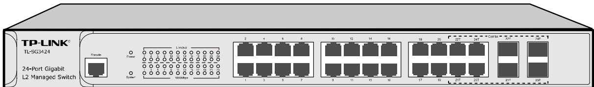
图 2-1 TL-SG3424 的前面板
