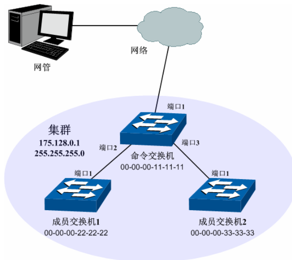
图 15-15 集群管理组网图
