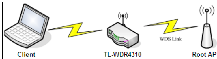
图 5-28 WDS 连接拓扑图
