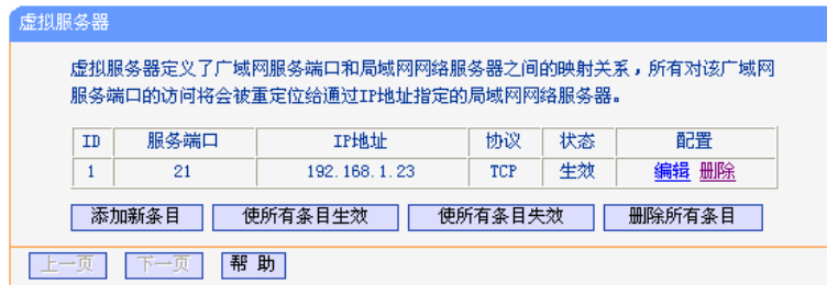
图 5-29 虚拟服务器
