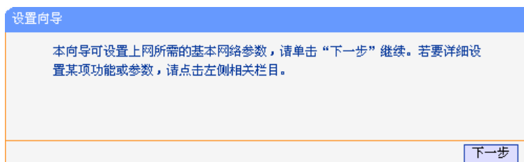
图 4-3 设置向导
