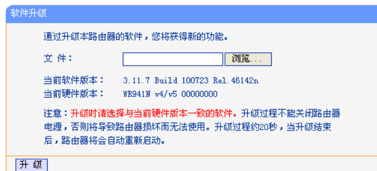
图 5-70 软件升级
