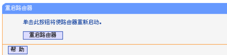
图 5-75 重启路由器
