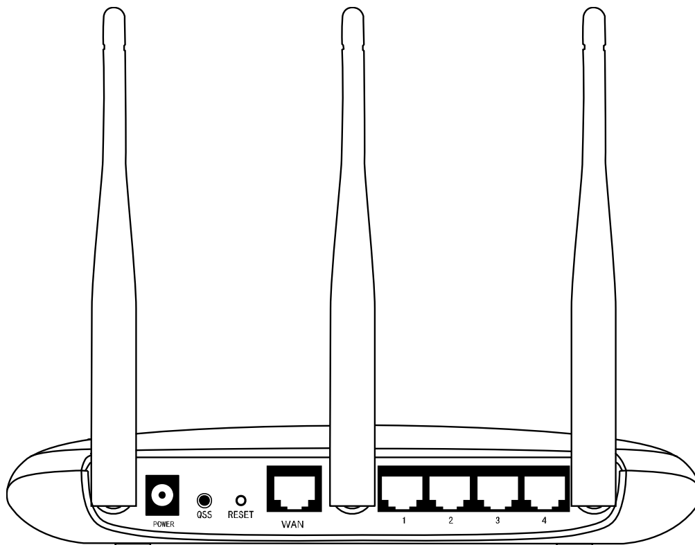
图 3-2 TL-WR941N 后面板示意图
