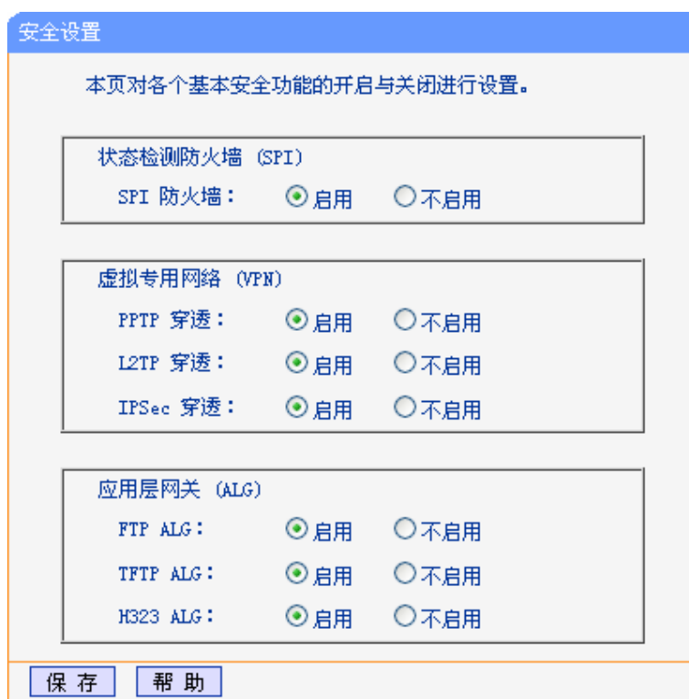
图 5-35 安全设置
