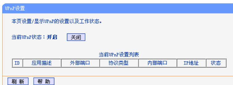
图 5-34 UPnP 设置
