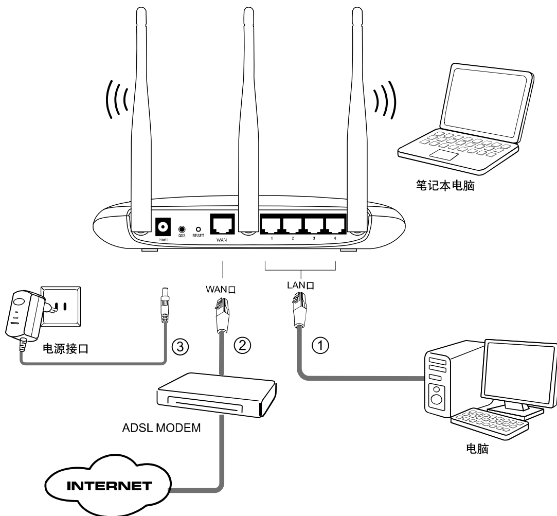
图 4-1 TL-WR941N 硬件安装示意图
