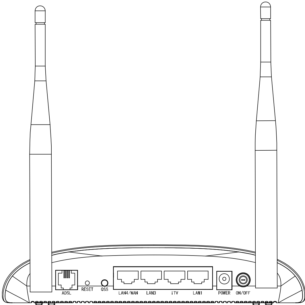
图 2 TD-W89841N 后面板示意图
