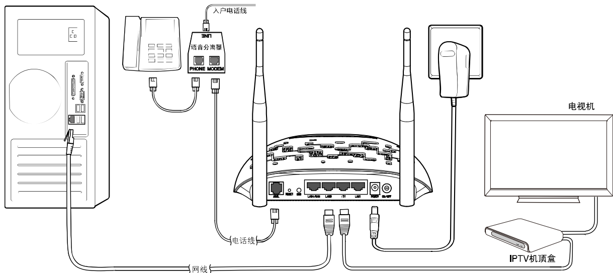
图 3 ADSL 宽带
