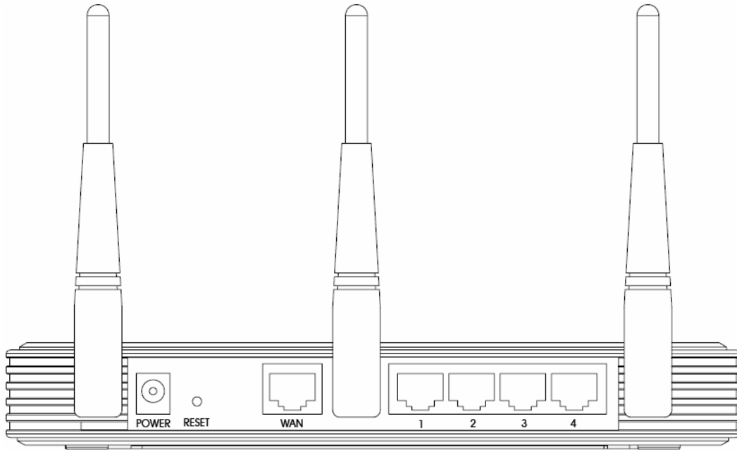
图 3-2 TL-WR941N 后面板示意图
