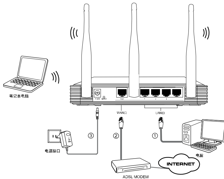
图 4-1 TL-WR941N 硬件安装示意图
