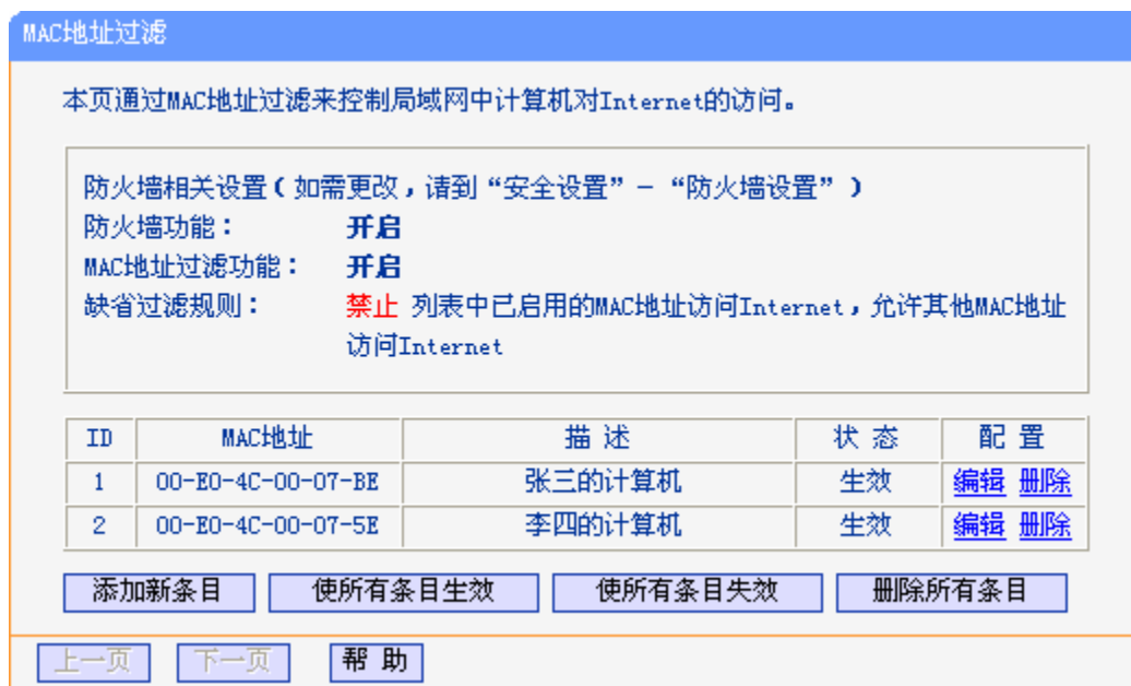
图 35 MAC 地址过滤
