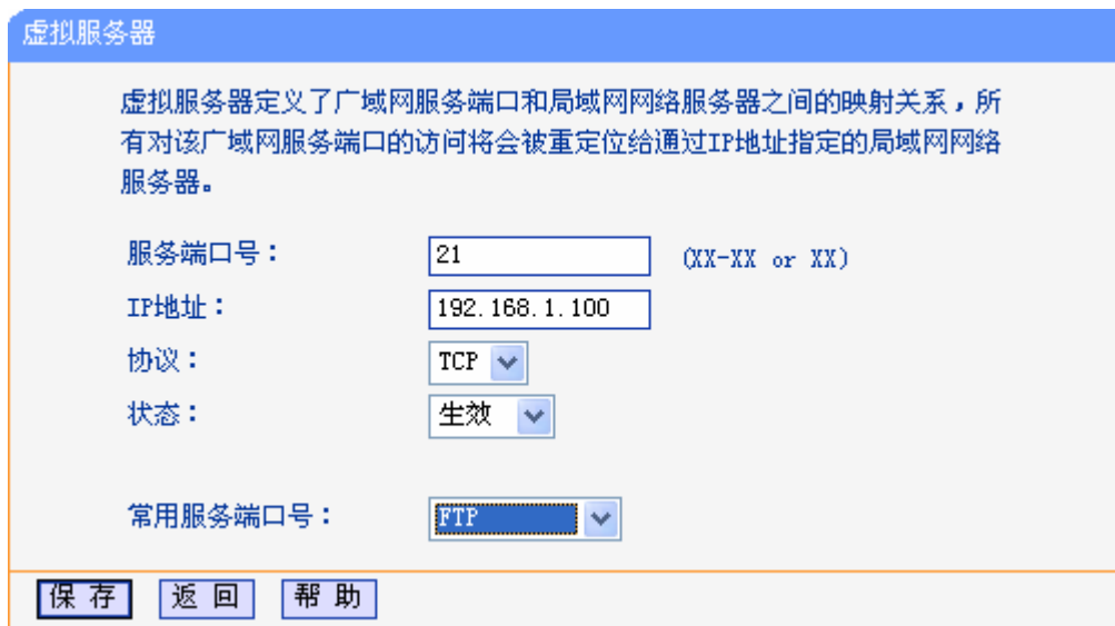
图 25 添加虚拟服务条目
