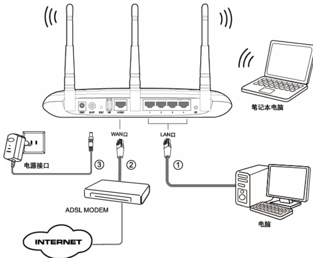
图 4-1 TL-WR2543N 硬件安装示意图
