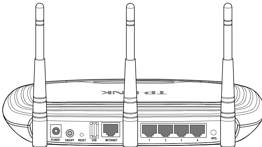
图 3-2 TL-WR2543N 后面板示意图
