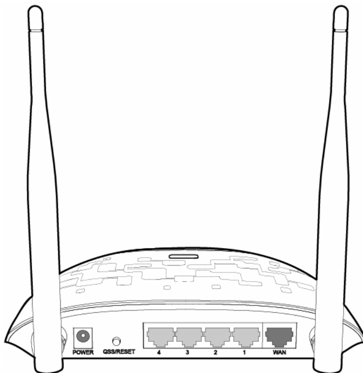
图 3-2 TL-WR843N 后面板示意图
