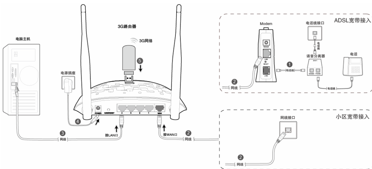
图 4-1 TL-WR843N 硬件安装示意图
