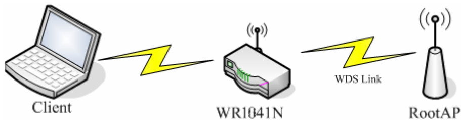
图 5-14 WDS 连接拓扑图
