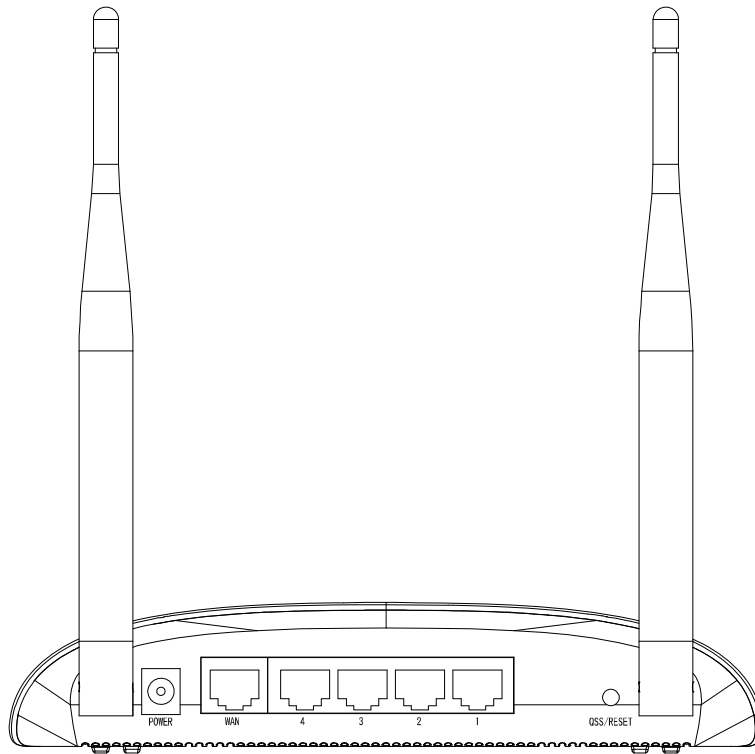
图 3-2 TL-WR1041N 后面板示意图
