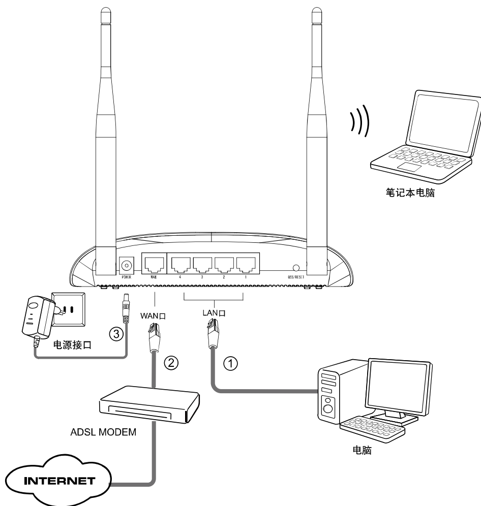
图 4-1 TL-WR1041N 硬件安装示意图
