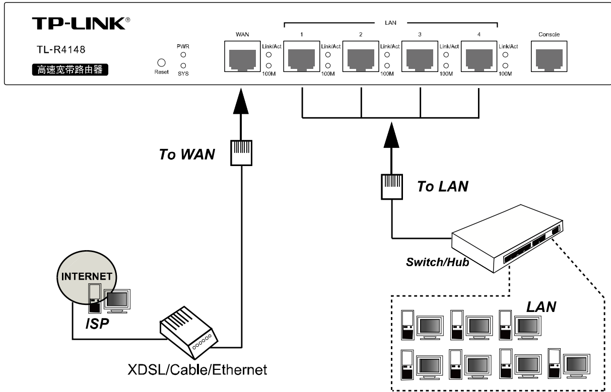
图 3.7 建立局域网和广域网连接
