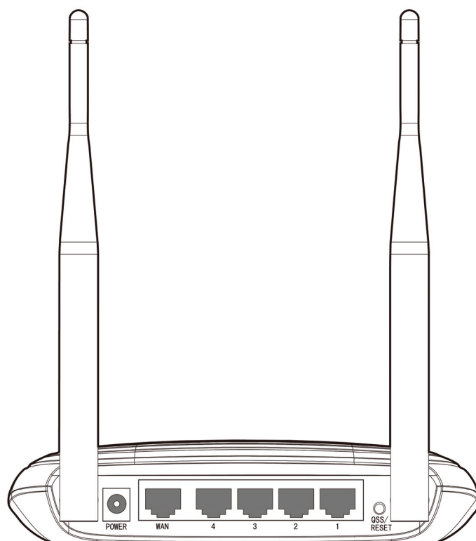
图 3-2 TL-WR840N 后面板示意图
