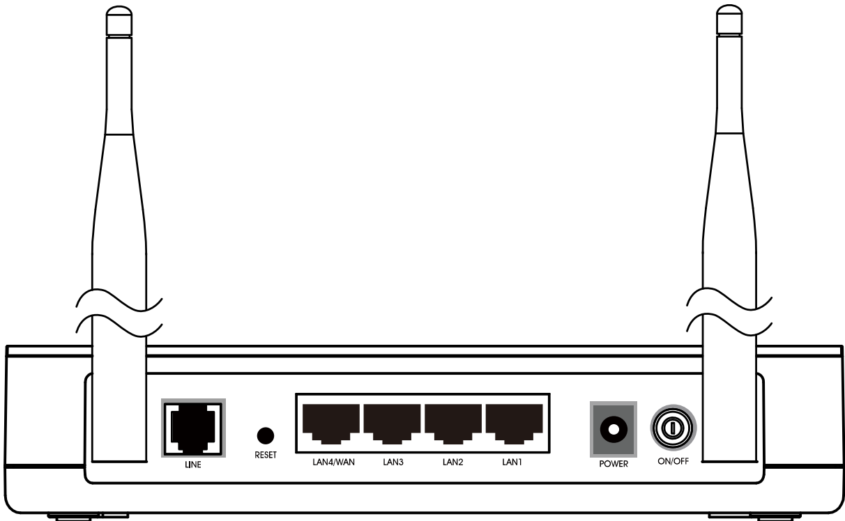
图 2 TD-W89841N 后面板示意图
