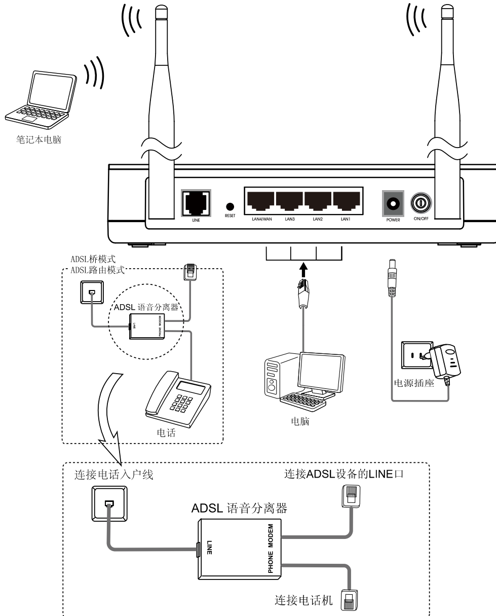
图3 TD-W89841N 硬件安装示意图
