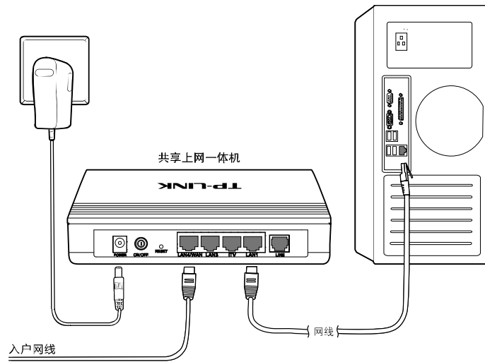
图 2-4 硬件连接图
