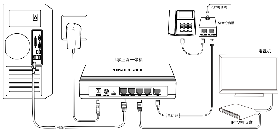
图 2-3 硬件连接图
