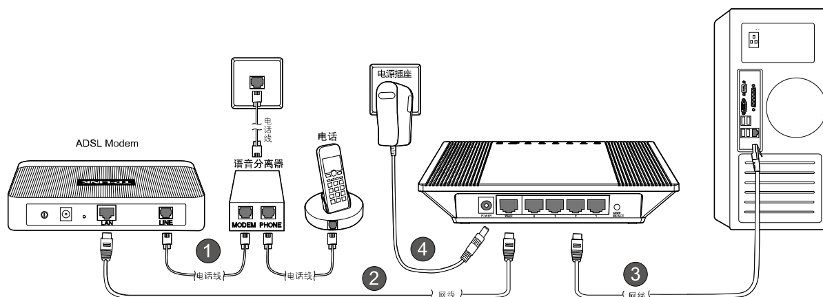
图 4-1 TL-WR746N 硬件安装示意图
