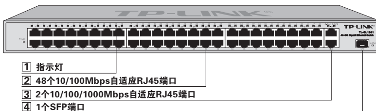
图1-1 TL-SL1351交换机前面板示意图
