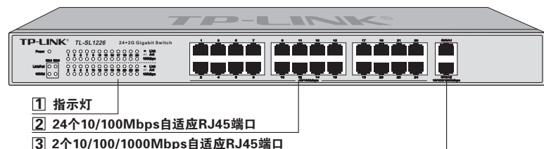
图1-2 TL-SL1226交换机前面板示意图
