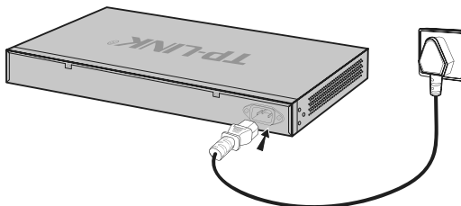
图3-2 电源线连接示意图
