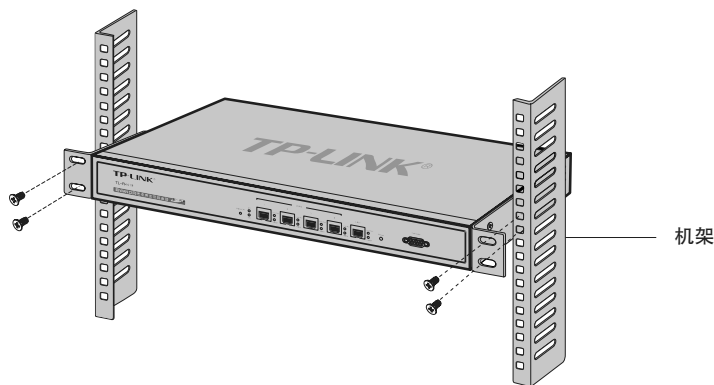
图2-3 机架安装示意图
