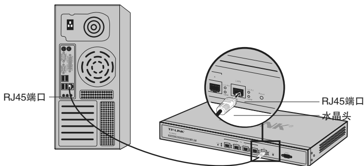
图3-1 RJ45端口连接示意图
