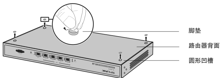
图2-1 桌面安装示意图
