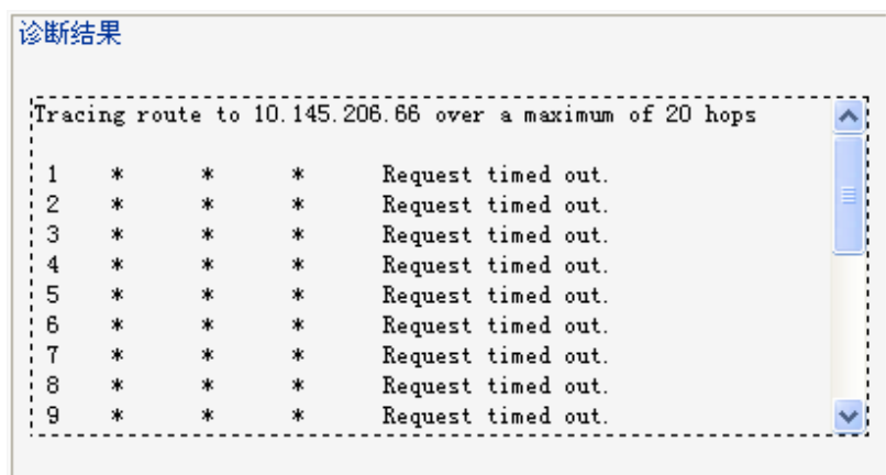
图 5-68 Tracert 诊断结果—失败
