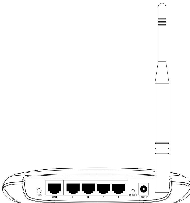
图 3-2 TL-WR741N 后面板示意图
