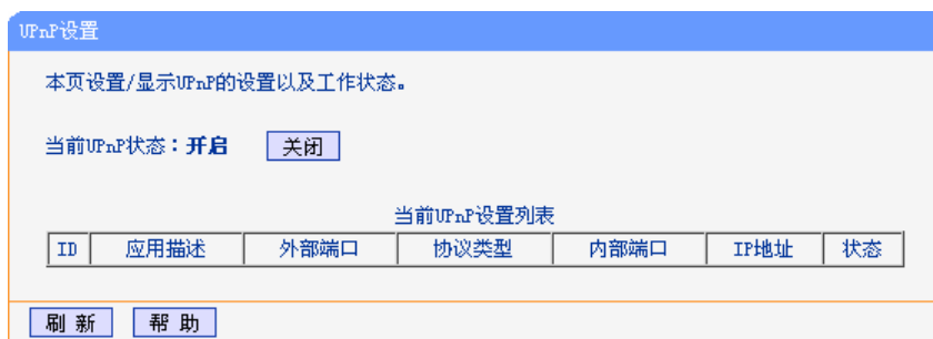
图 5-32 UPnP 设置
