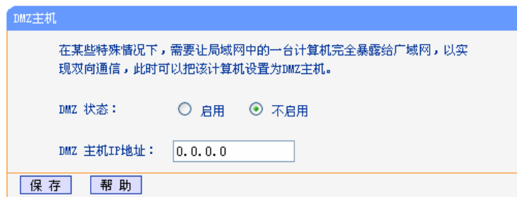
图 5-31 DMZ 主机
