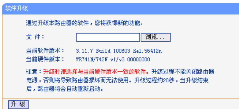
图 5-69 软件升级
