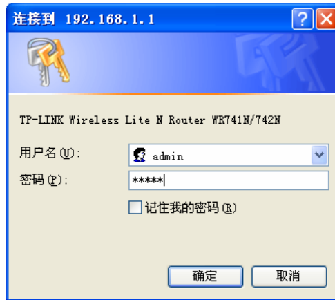
图 4-2 登录界面
