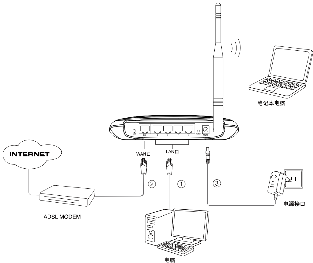
图 4-1 TL-WR741N/TL-WR742N 硬件安装示意图
