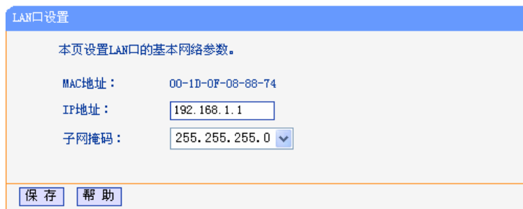
图 5-3 LAN 口设置
