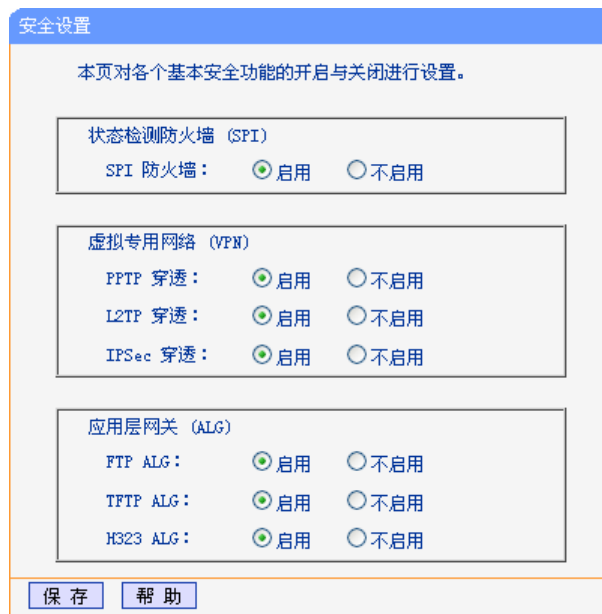
图 5-33 安全设置
