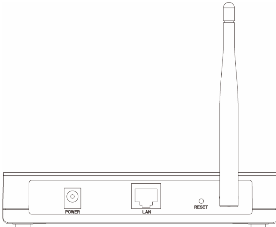
图 2-2 TL-WA701N 后面板示意图
