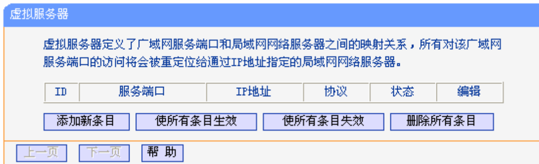
图 25 虚拟服务器
