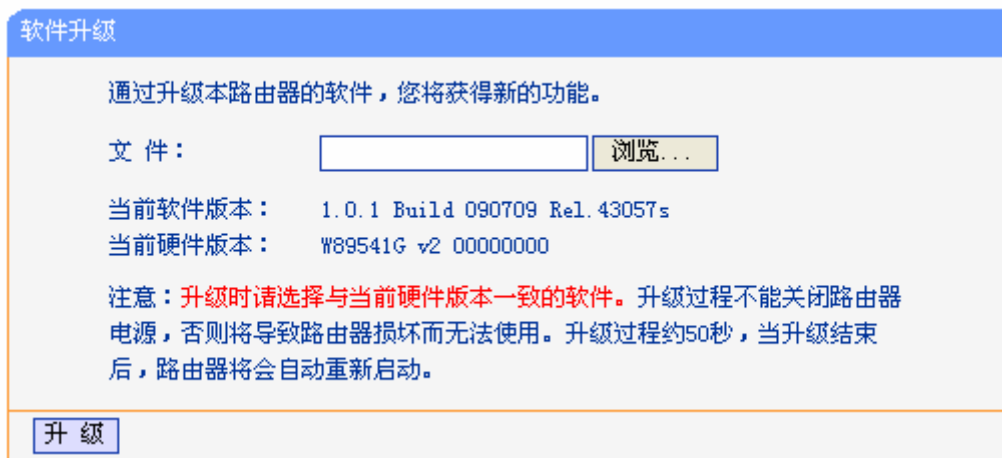
图 49 软件升级
