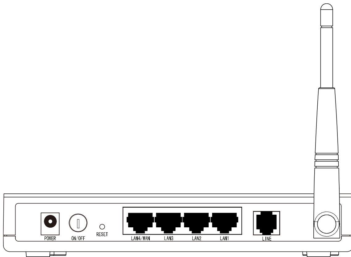
图 2 TD-W89541G 系列后面板示意图
