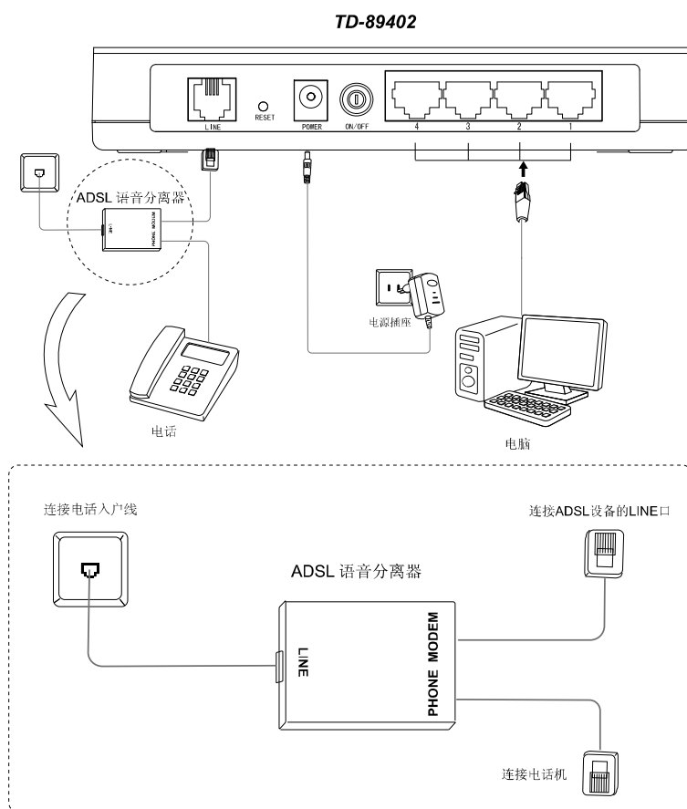
图3 硬件连接图
