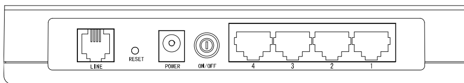
图 2 TD-89402 后面板示意图
